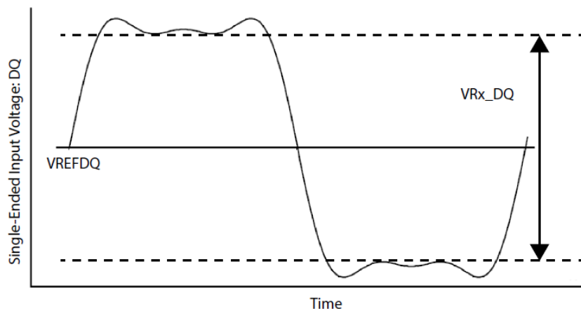
Figure 24. VR x _DQ
