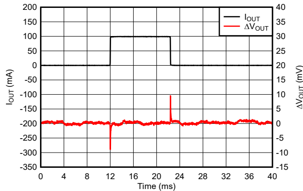
图 5-43. TPS76933 负载瞬态响应 (新芯片)
