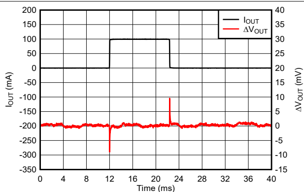
图 7-16. TPS76933 负载瞬态响应 (新芯片)
