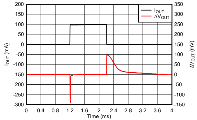
图 5-44. TPS76933 负载瞬态响应 (新芯片)
