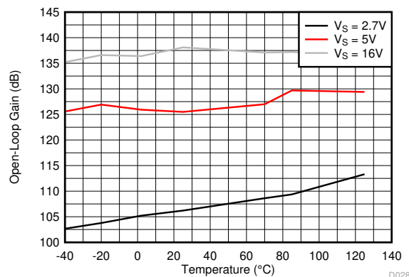
图 5-29. 开环电压增益与温度间的关系 (dB)
