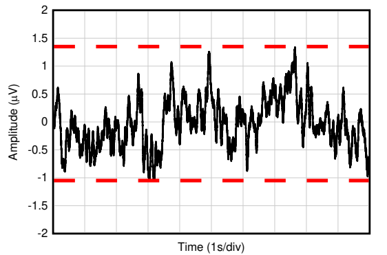
图 5-25. 0.1Hz 至 10Hz 噪声
