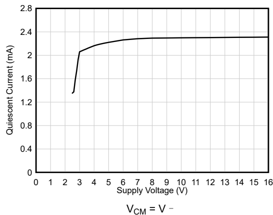
图 5-27. 静态电流与电源电压间的关系
