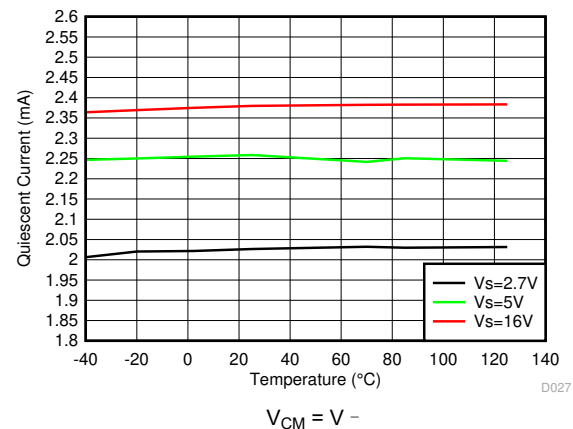
图 5-28. 静态电流与温度间的关系
