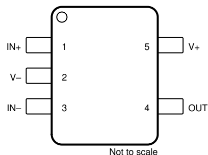
图 4-2. TLV9161 DCK 封装 5 引脚 SC70 (顶视图)
