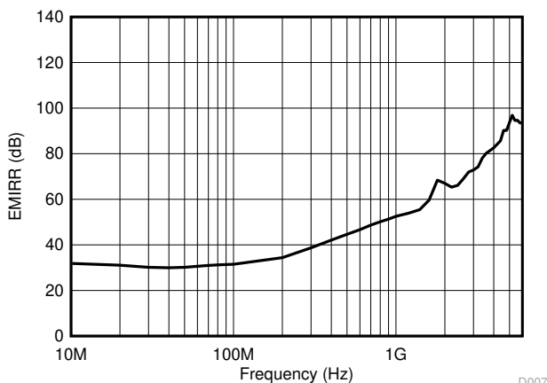
图 7-1. EMIRR Testing
