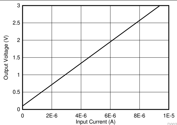
图 9-5. 光电二极管放大器电路直流结果
