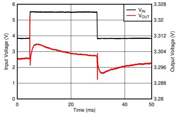
图 5-8. Line Transient
