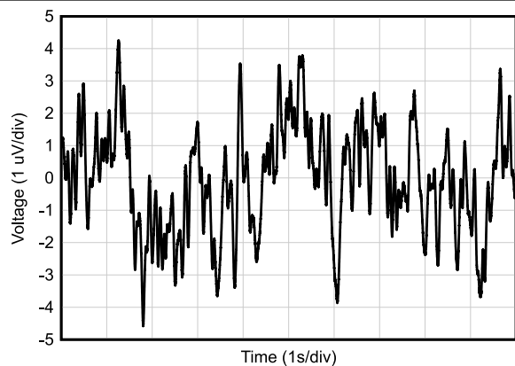
图 5-17. 0.1-Hz to 10-Hz Noise
