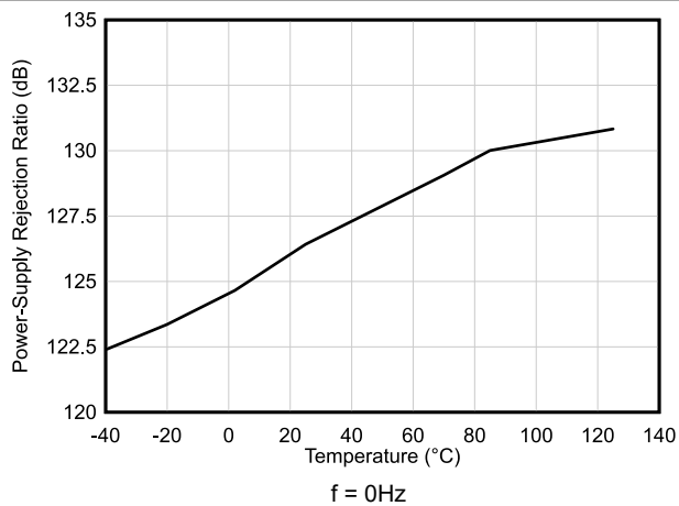
图 5-16. PSRR vs Temperature (dB)
