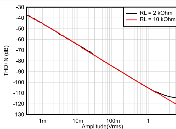
图 5-20. THD+N vs Output Amplitude
