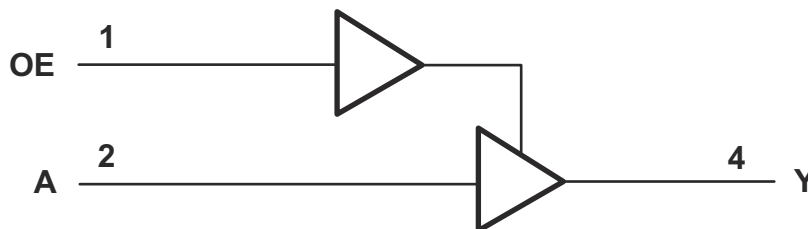
图 8-1. Logic Diagram
