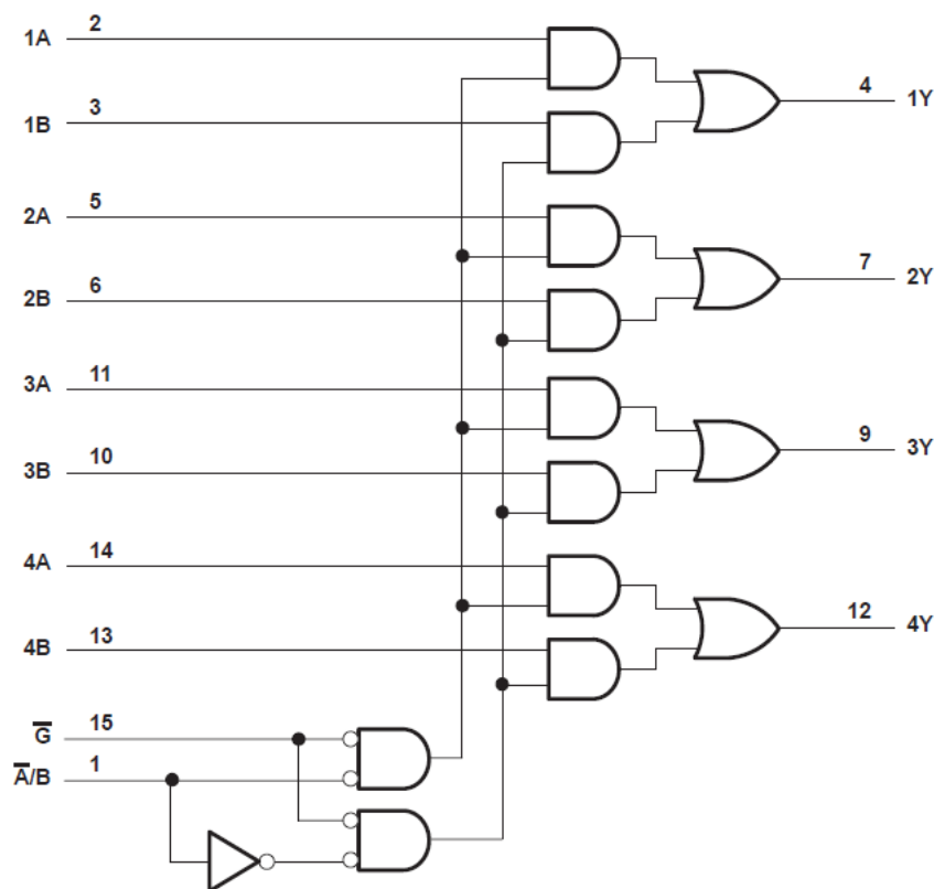
功能方框图
