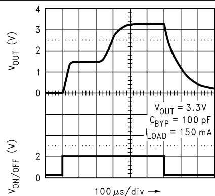
图 5-51. Turn-On Time (Legacy Chip)
