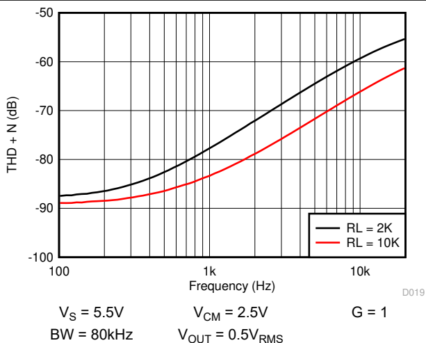
图 6-13. THD+N 与频率间的关系
