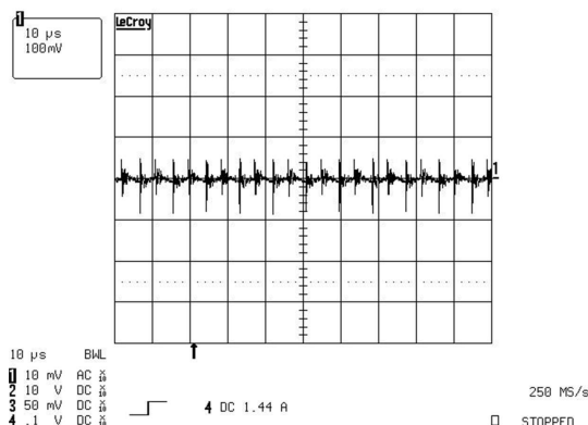
图 8-11. 满载条件下的输出电压纹波 (100mV/div)
