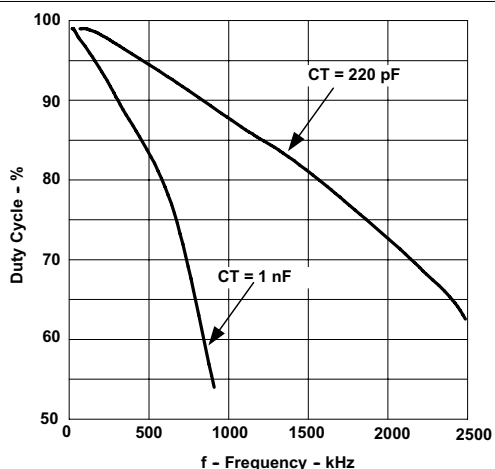
图 6-15. 最大占空比与振荡器频率间的关系
