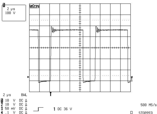
图 8-8. 240V 交流输入下的初级侧 MOSFET 漏源电压 (100V/div)
