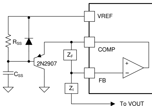
图 7-6. 软启动实现
