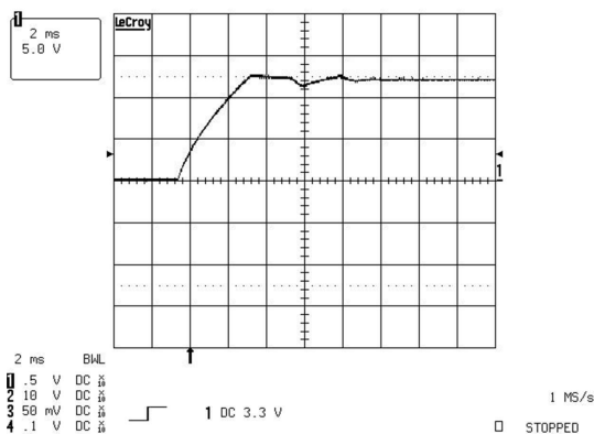
图 8-12. 满载启动条件下的输出电压行为 (5V/div)
