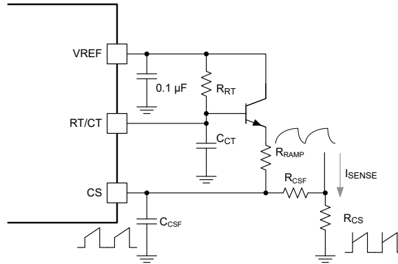
图 7-8. 斜率补偿电路
