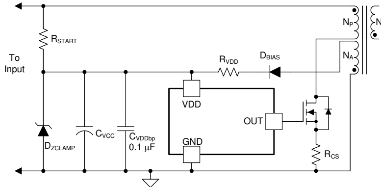
图 7-1. VDD 保护
