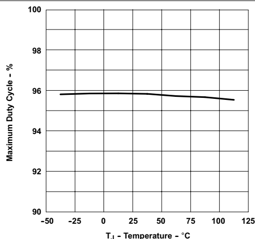
图 6-16. 最大占空比与温度间的关系 (对于具有最大 100% 占空比的器件型号)
