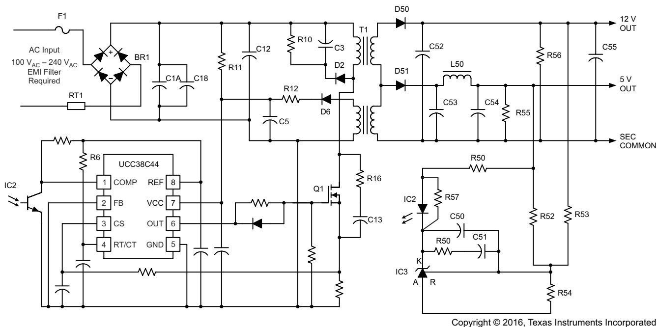
图 8-1. 典型的离线应用
