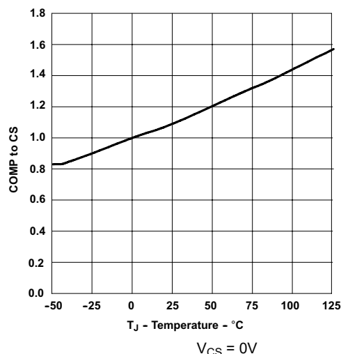
图 6-4. COMP 至 CS 失调电压与温度间的关系
