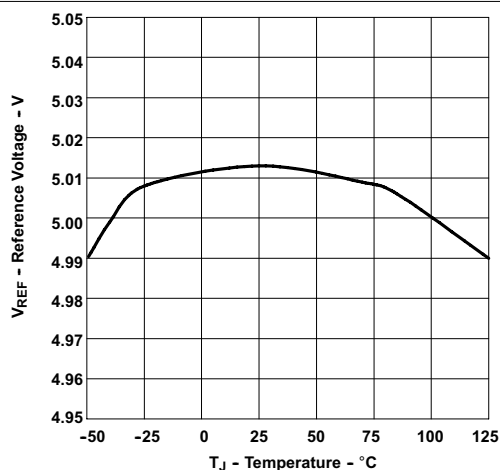
图 6-5. 基准电压与温度间的关系
