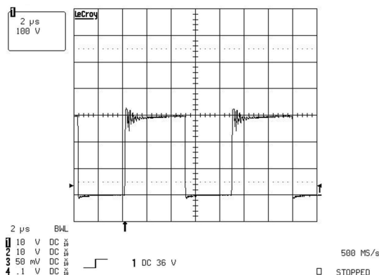
图 8-9. 120V 交流输入下的初级侧 MOSFET 漏源电压 (100V/div)
