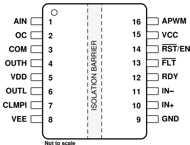
图 4-1. UCC21710-Q1 DW SOIC (16) Top View
