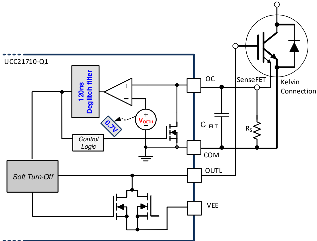
图 7-6. Soft Turn-off
