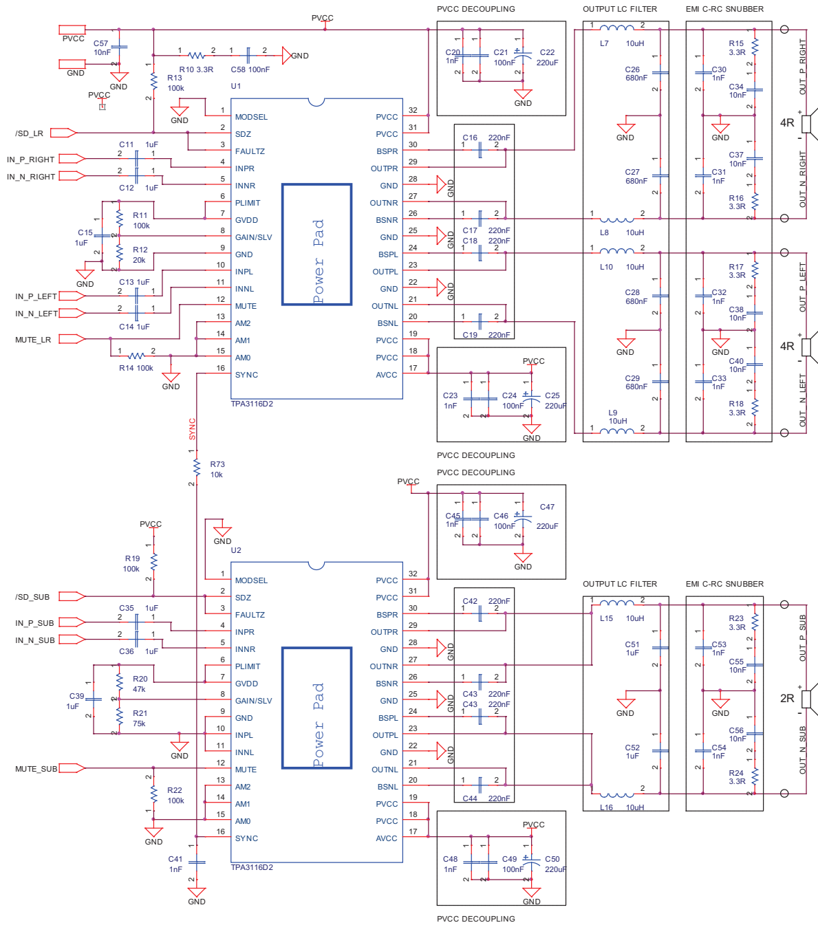
图 37. Schematic
