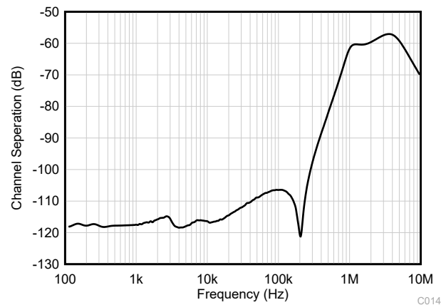
图 6-40. 通道隔离与频率间的关系
