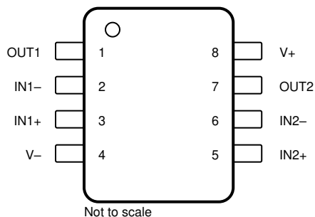
图 5-3. TLV9352 D、DDF、DGK 和 PW 封装 8 引脚 SOIC、SOT-23、TSSOP 和 VSSOP ( 顶视图 )
