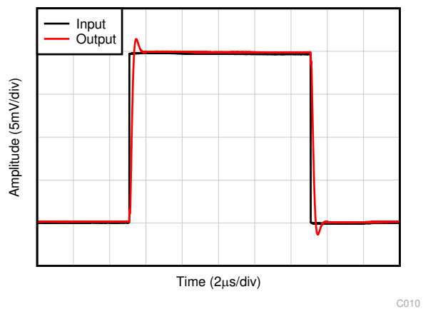
图 6-33. 正过载恢复
