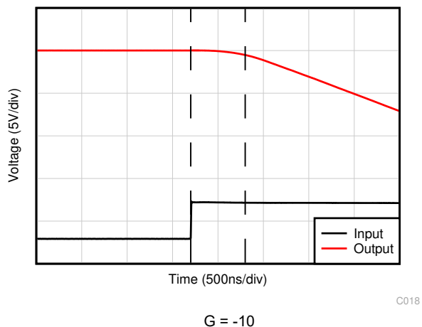
图 6-33. 正过载恢复
