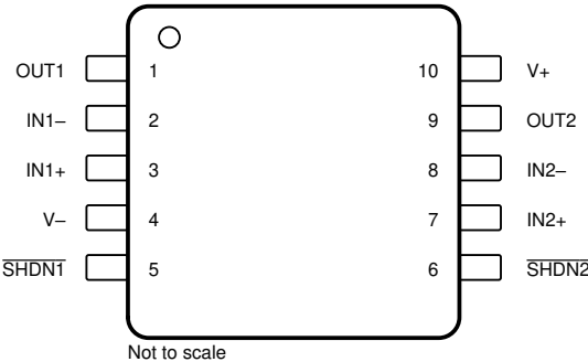
图 4-8. TLV9062S DGS 封装，10 引脚 VSSOP（顶视图）
