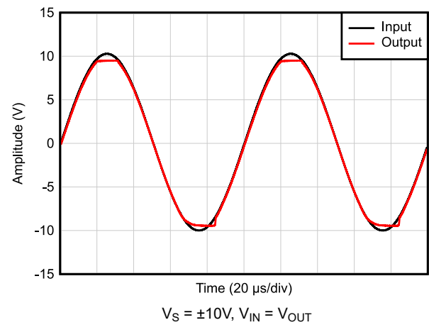
图 5-28. No Phase Reversal
