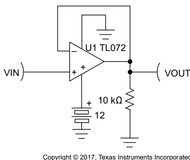
图 9-3. 单电源单位增益放大器
