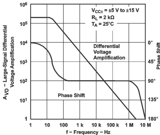
图 6-48. 大信号差分电压放大和相移与频率间的关系
