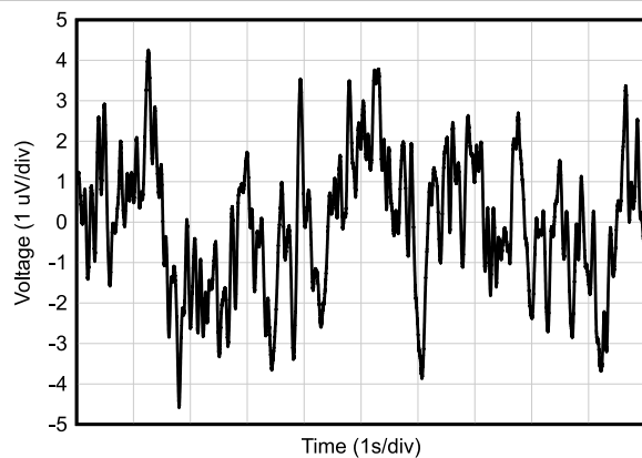
图 6-17. 0.1Hz 至 10Hz 噪声
