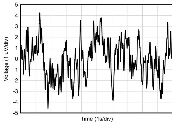
图 6-17. 0.1Hz 至 10Hz 噪声
