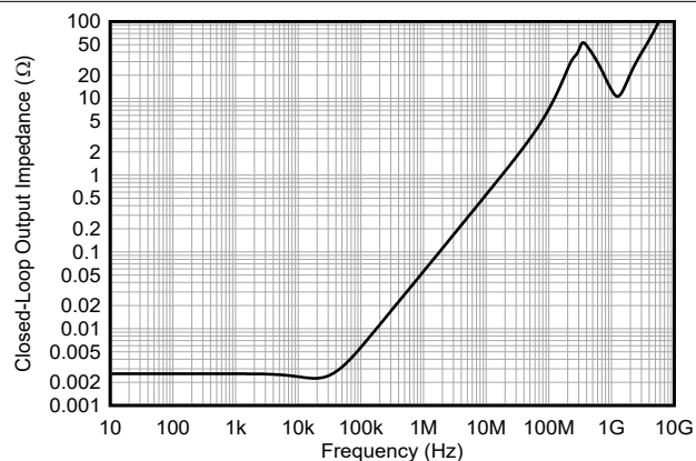
图 6-30. 输出阻抗与频率间的关系
