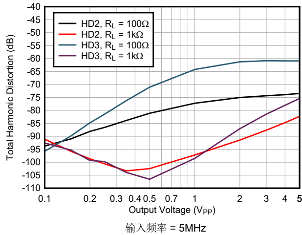
图 6-9. 谐波失真与输出电压摆幅间的关系
