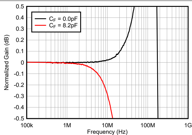
图 6-1. 小信号频率响应
