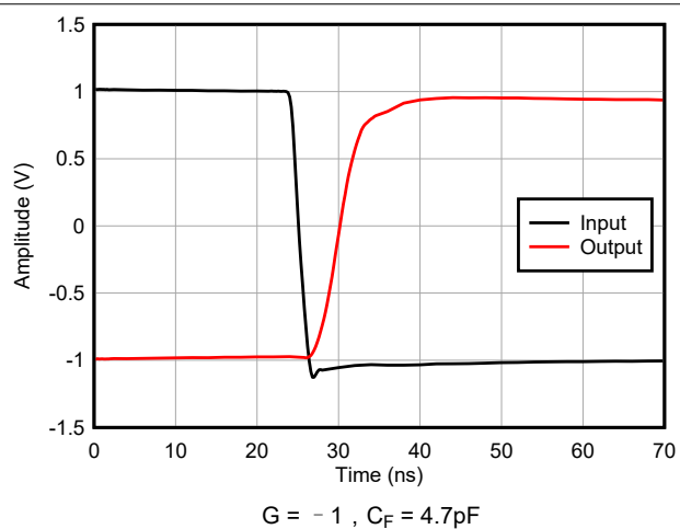
图 6-24. 趋稳时间
