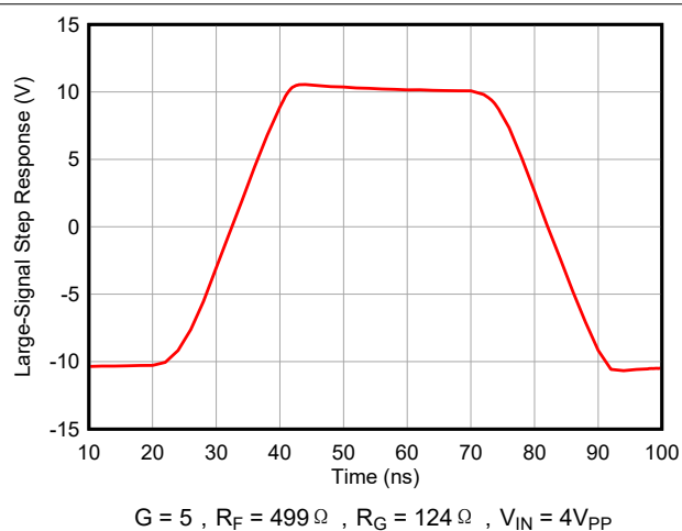
图 6-23. 大信号瞬态响应
