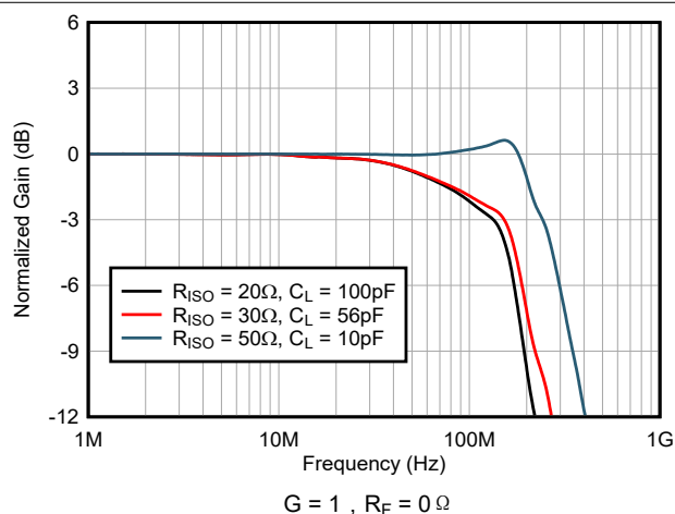
图 6-6. 频率响应与容性负载间的关系
