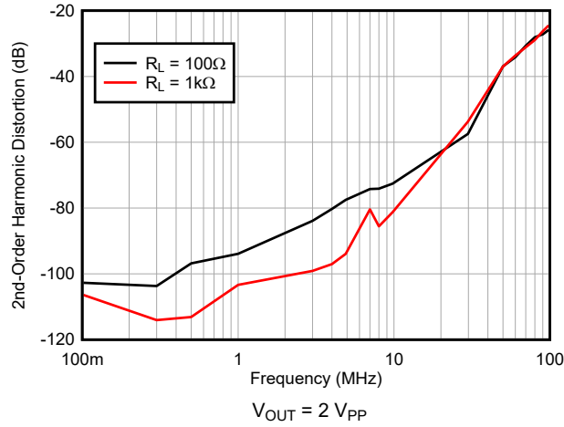
图 6-7. 第二谐波失真与频率间的关系
