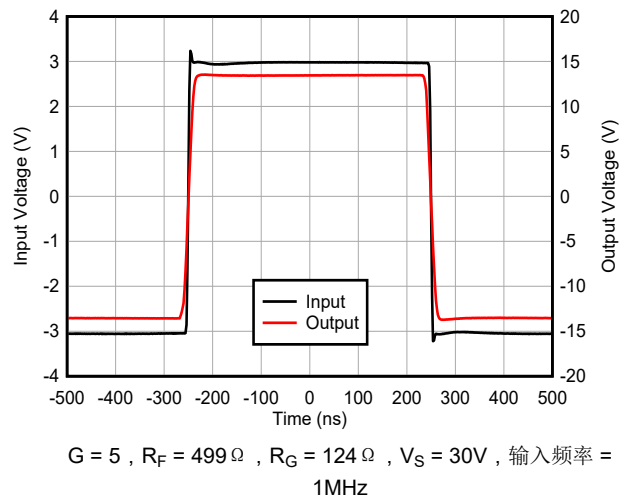
图 6-28. 过驱恢复
