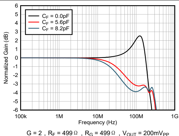
图 6-2. 小信号频率响应
