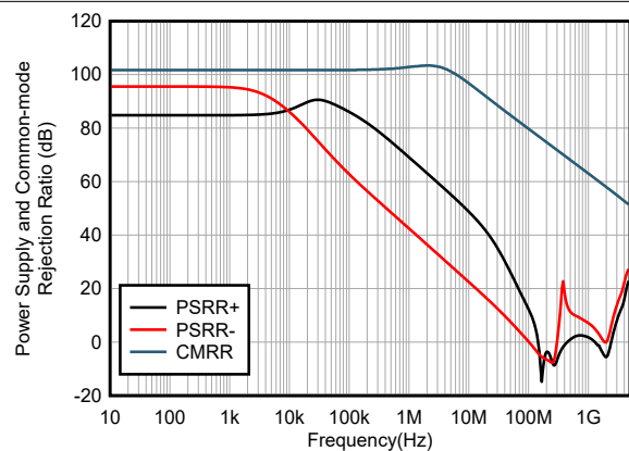
图 6-29. 抑制比与频率间的关系
