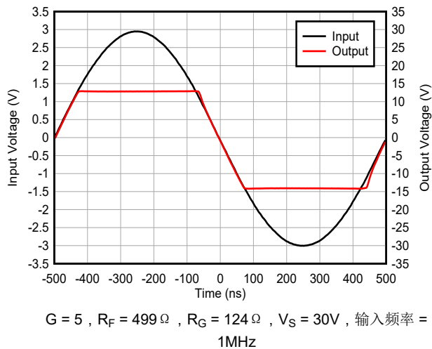
图 6-27. 过驱恢复
