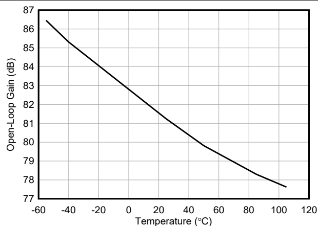
图 6-13. 开环增益与温度间的关系
