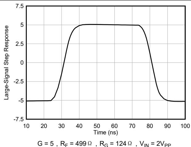
图 6-22. 大信号瞬态响应
