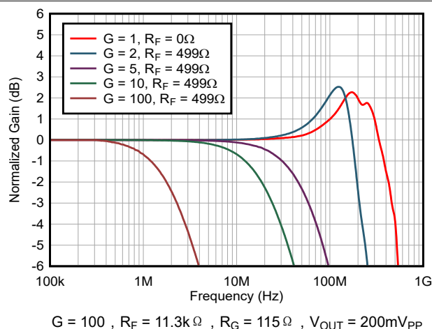
图 6-1. 小信号频率响应
