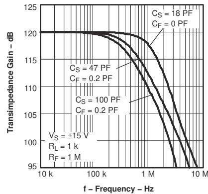
图 8-8. 1M \Omega 互阻抗响应
