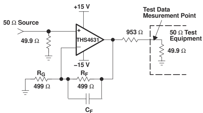
图 7-1. 交流测量配置
