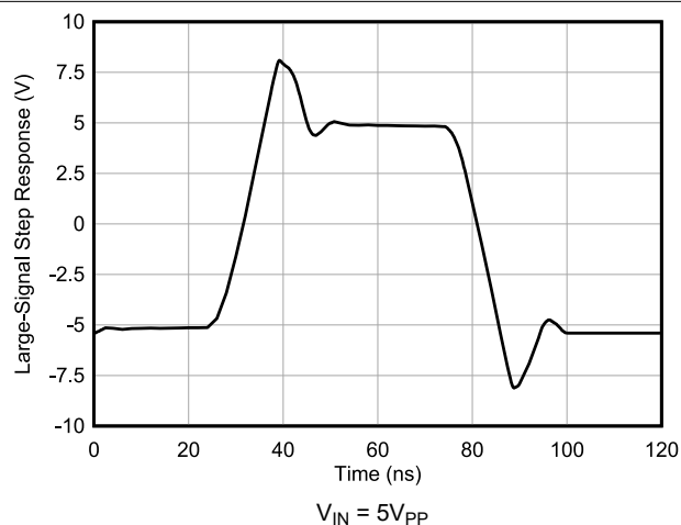
图 6-21. 大信号瞬态响应
