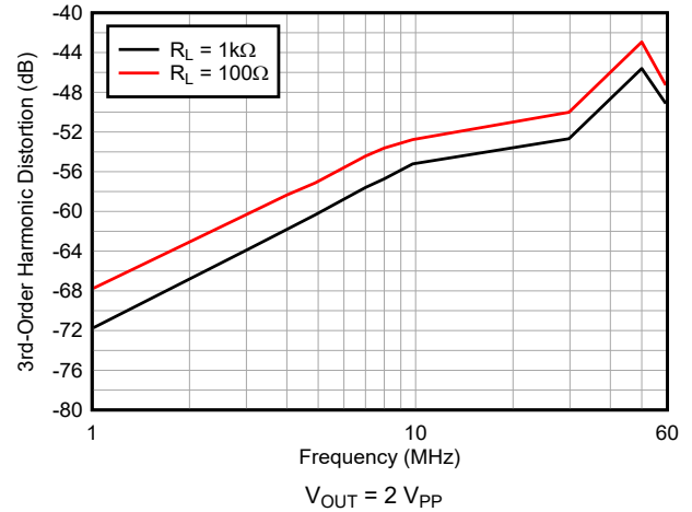
图 6-8. 第三谐波失真与频率间的关系
