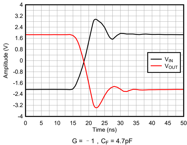
图 6-25. 趋稳时间
