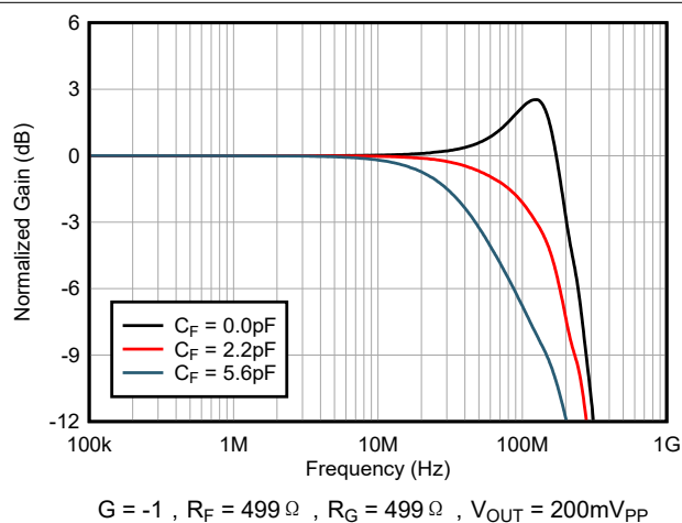
图 6-4. 小信号频率响应
