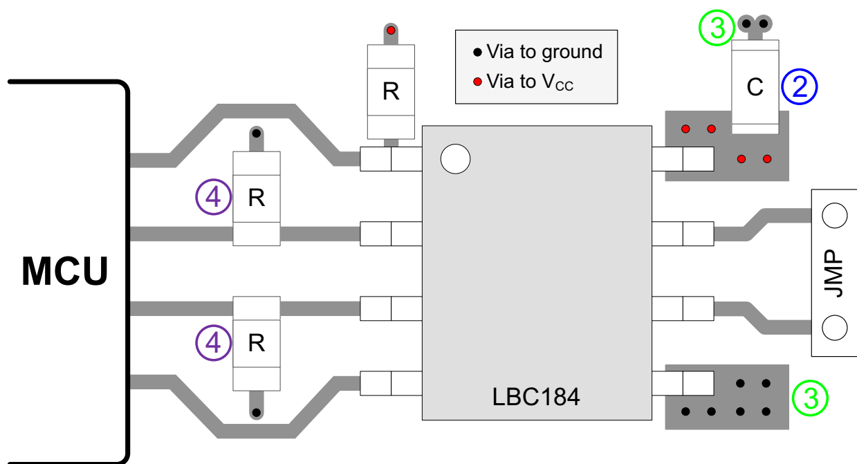
图 8-7. Layout Schematic
