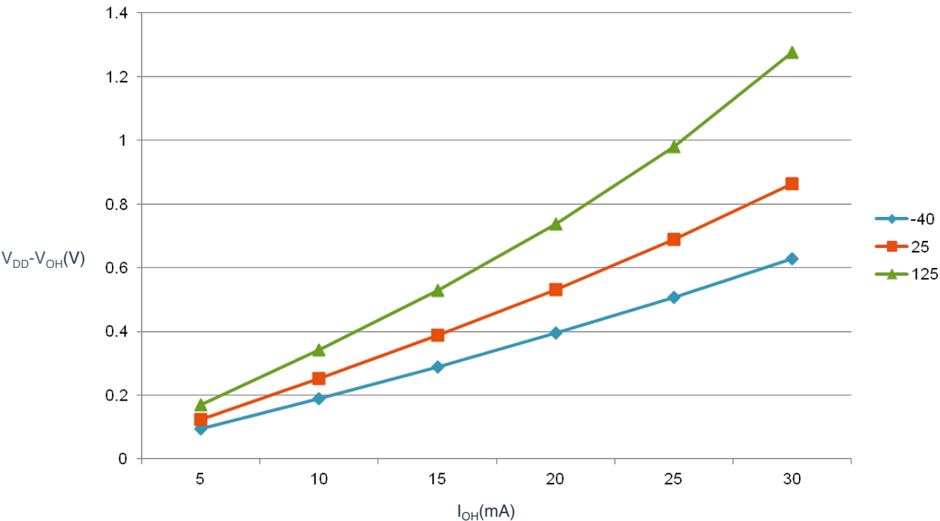
图 4. 典型 V_{DD}-V_{OH} 对比 I_{OH} (高驱动强度) ( V_{DD} = 3\text{ V} )
