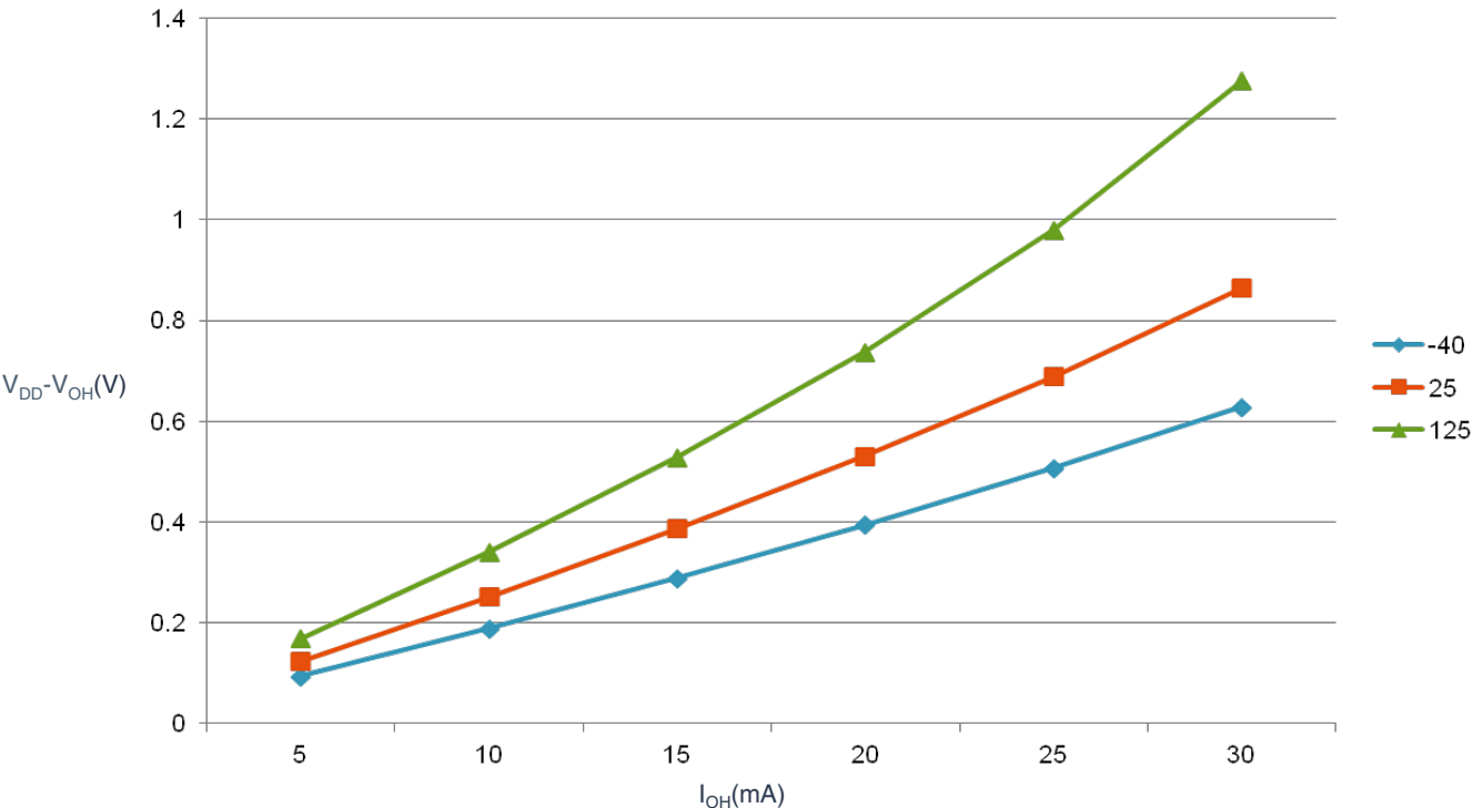
图 3. 典型 V_{DD}-V_{OH} 对比 I_{OH} (高驱动强度) ( V_{DD} = 5\text{ V} )
