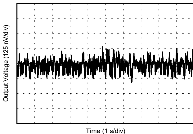
图 6-5. 0.1Hz 至 10Hz 噪声
