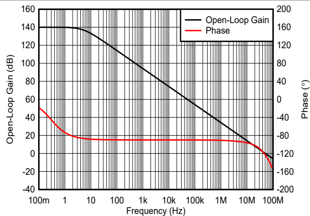
图 6-24. 开环增益和相位与频率间的关系
