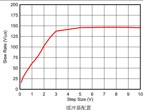
图 6-39. 压摆率与输出阶跃大小间的关系
