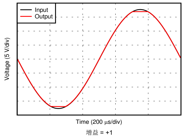
图 6-30. 无相位反转
