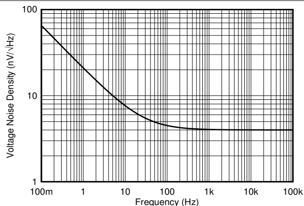
图 6-1. 输入电压噪声密度与频率间的关系
