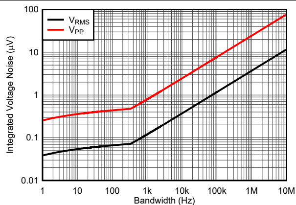
图 6-2. 集成输入电压噪声与带宽间的关系
