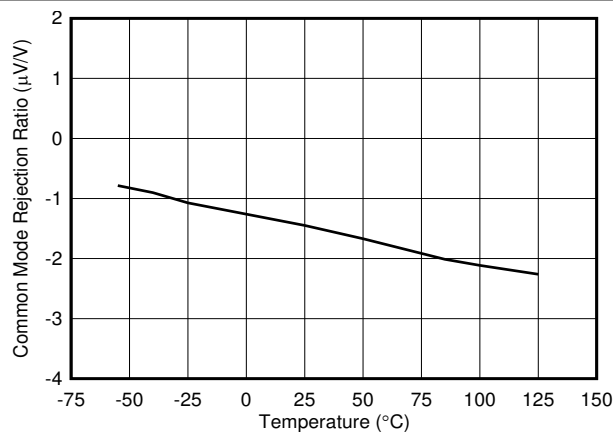
图 6-23. 共模抑制比与温度间的关系
