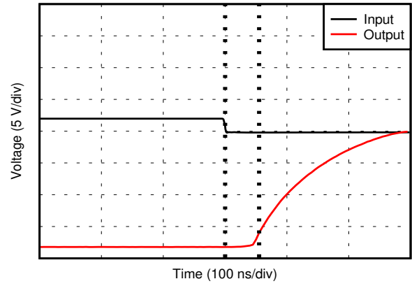
图 6-30. 无相位反转
