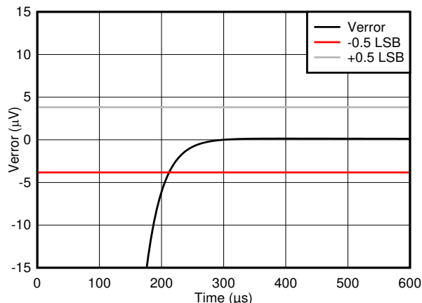
图 8-2. OPA828 输出稳定时间
