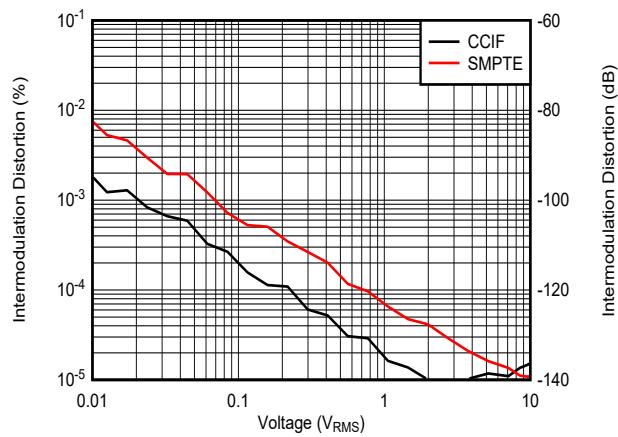
图 6-41. 互调失真
