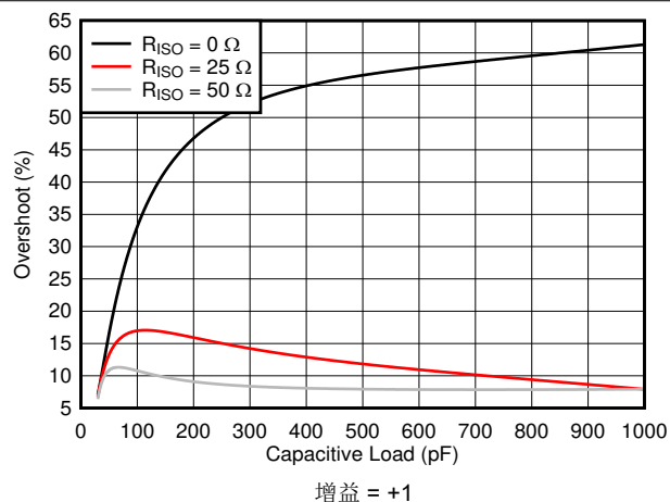
图 6-28. 小信号过冲与容性负载间的关系
