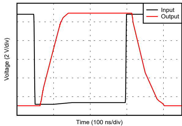
图 6-32. 负过载恢复
