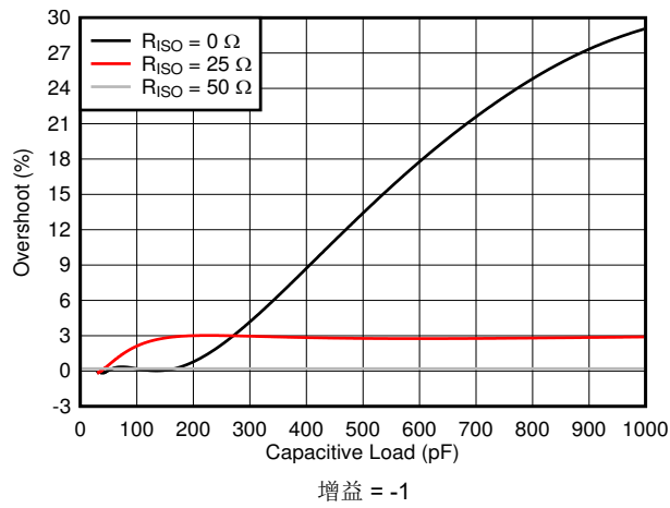
图 6-29. 小信号过冲与容性负载间的关系
