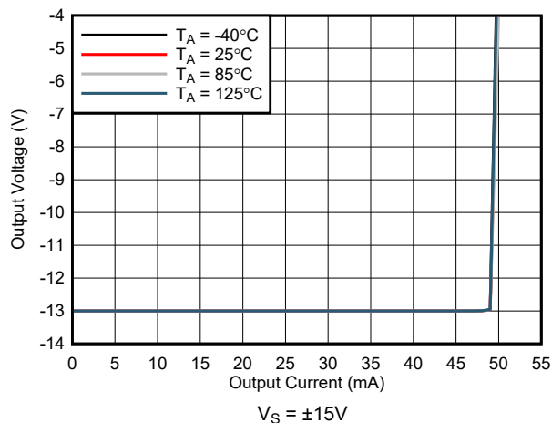
图 6-19. 输出电压摆幅与输出灌电流间的关系
