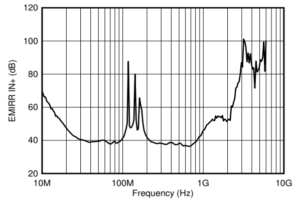
图 6-42. 电磁干扰抑制
