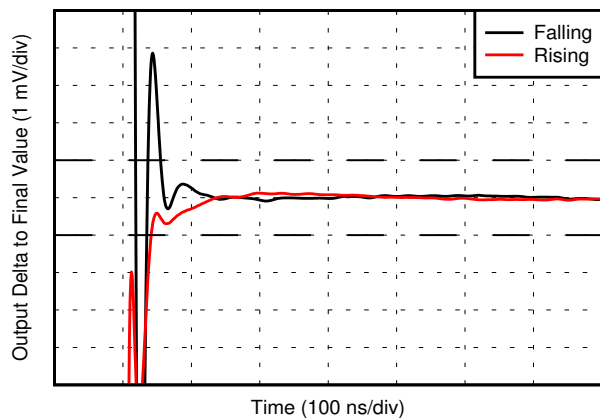
图 6-35. 12 位稳定时间
