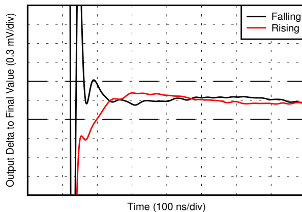
图 6-36. 14 位稳定时间
