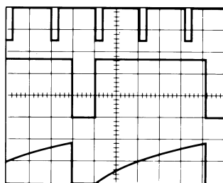
图 8-4. 分频器波形
