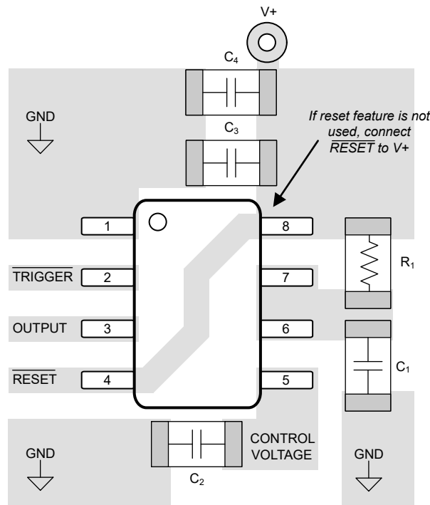
图 8-10. PCB 布局
