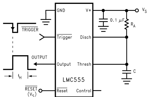
图 8-3. 单稳 (一次性)
