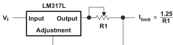
图 7-5. 精密限流电路
