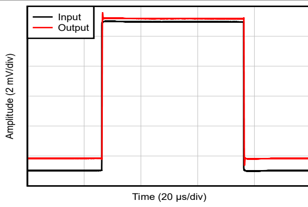
图 5-26. 小信号阶跃响应, G = 1
