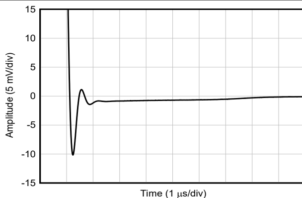
图 5-28. 大信号阶跃响应 (下降)
