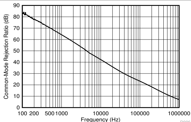
图 5-39. 共模抑制比
