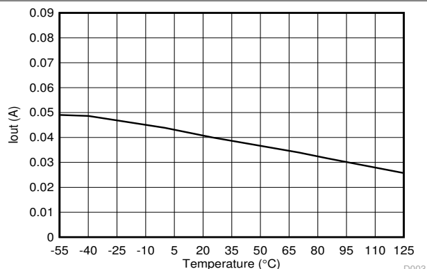
图 5-37. 拉电流限制
