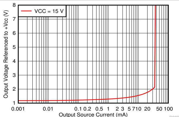
图 5-36. 输出拉电流特性
