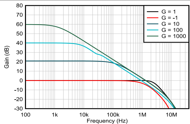
图 5-6. 闭环增益与频率间的关系
