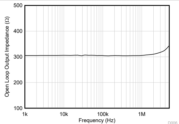
图 5-24. 开环输出阻抗与频率间的关系
