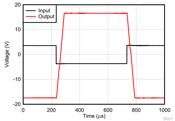
G = -10 图 5-28. 过载恢复
