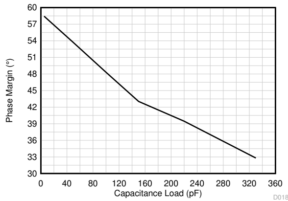
图 5-27. 相位裕度与容性负载间的关系
