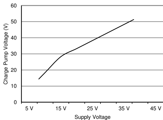
图 6-3. V_{CP} vs V_{BB}
