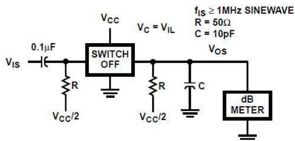
图 15-4. 关闭信号馈通测试电路
