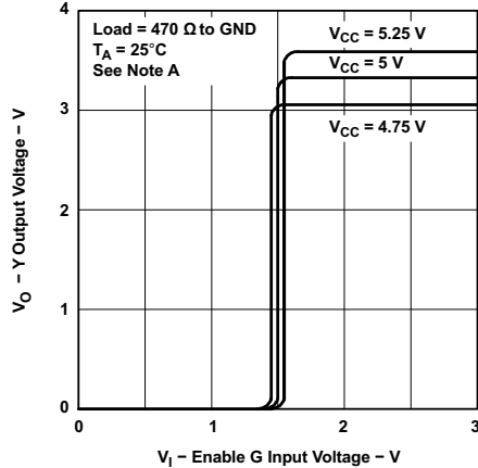
图 5-1. Output Voltage vs Enable G Input Voltage
